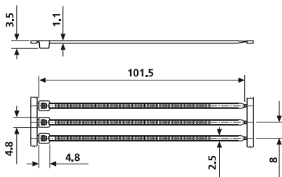
Bandoleer T18RA
