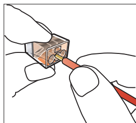
Die Doppelfeder ermöglicht leichtes Stecken des Leiters.
